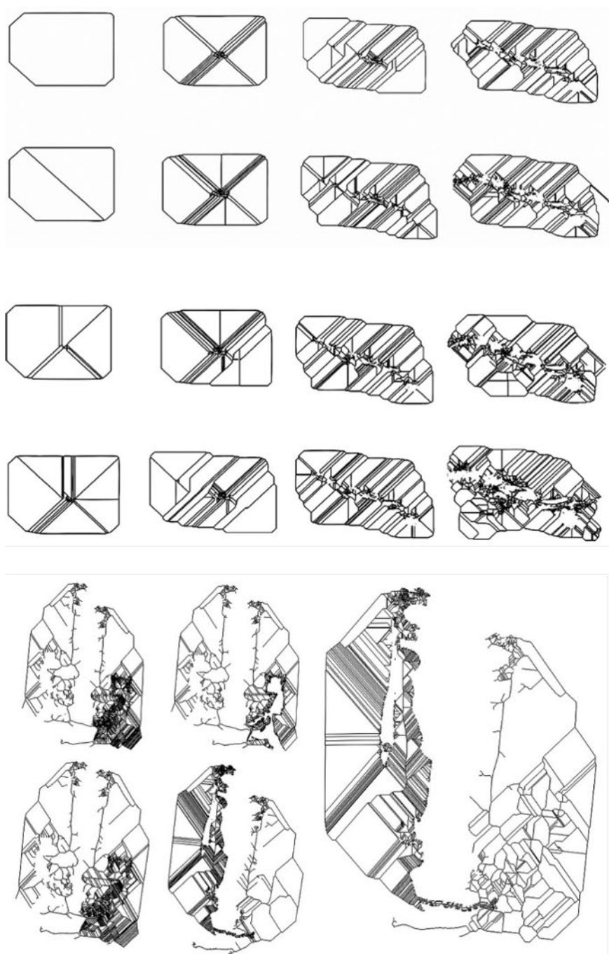
Figura 6. Trama generada en software LSVG (sistemas iterados)
