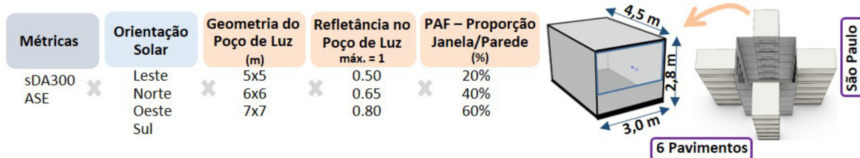
Figura 1. Configurações dos modelos simulados
