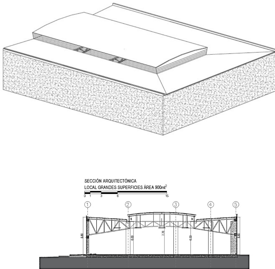
Figura 3. Esquema volumétrico y sección transversal del local objeto de estudio
