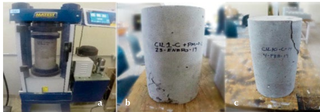
Figura 3. a) Prensa; b) Mezcla de polvo de mármol; c) Mezcla normal. Fuente: Rubio Sánchez (2019).
