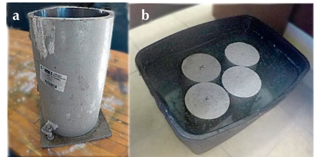
Figura 2. a) Molde cilindro; b) Curado de cilindros. Fuente: Rubio Sánchez (2019).
